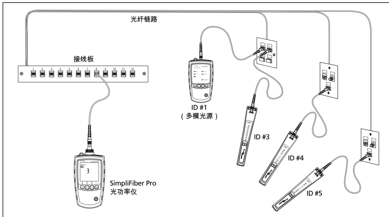
图 6. 使用 FindFiber 模式给光纤定位
