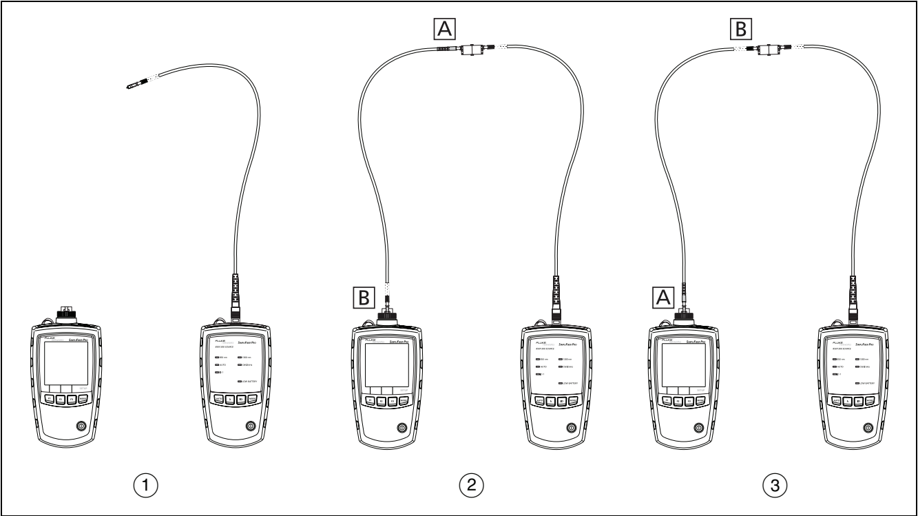
图 A-3. 用于测试测试基准线的连接
