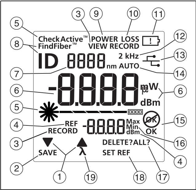
图 3. 显示屏功能
