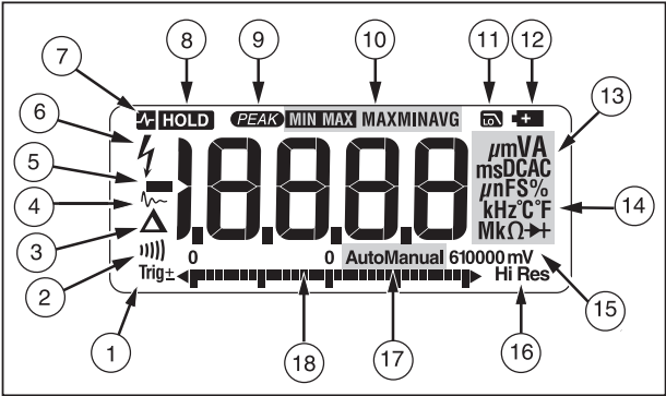
图 1. 显示屏特性
