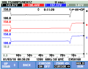
图 23-5. 趋势图显示（光标功能启用）
