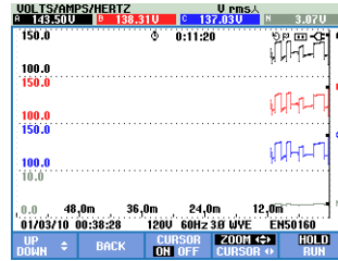
图 23-6. 趋势图显示（光标和缩放功能启用）
