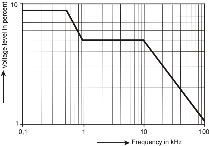
图 24-4. 依照 EN50160 标准的 Meister Kurve
