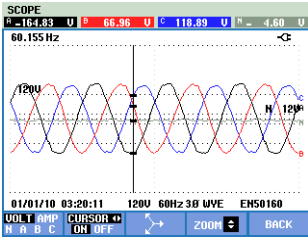
图 23-3. 波形显示（光标和缩放功能启用）
