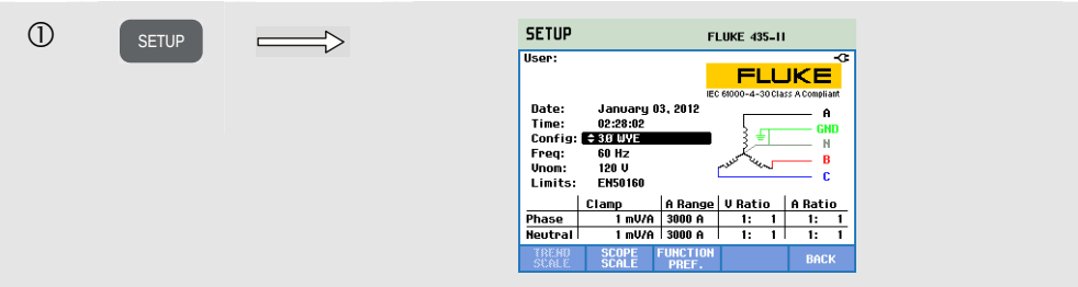
图 24-3. 屏幕显示实际接线配置
