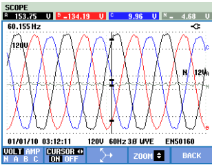
图 23-2. 波形显示（光标功能启用）
