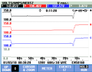
图 23-4. 趋势图显示（光标功能关闭）
