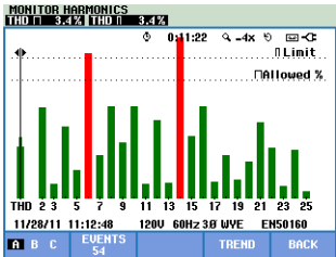
图 16-4. 条形图屏幕
