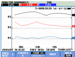
图 16-2. 趋势图显示
