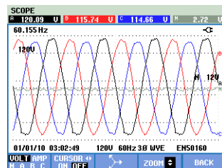
图 23-1. 波形显示（光标功能关闭）
